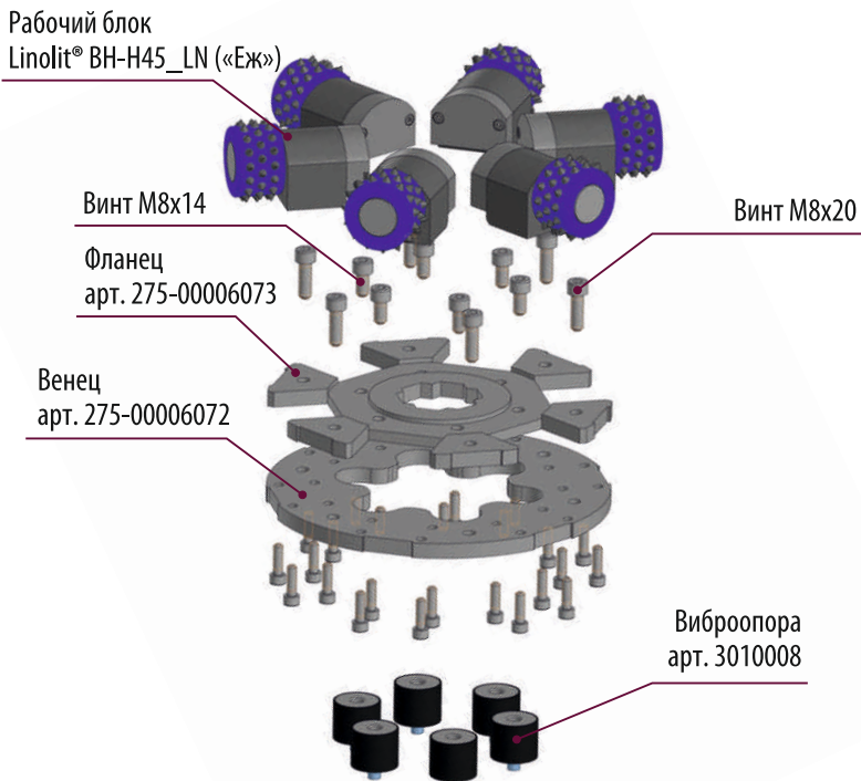
Рис. 10 Установка рабочих блоков
