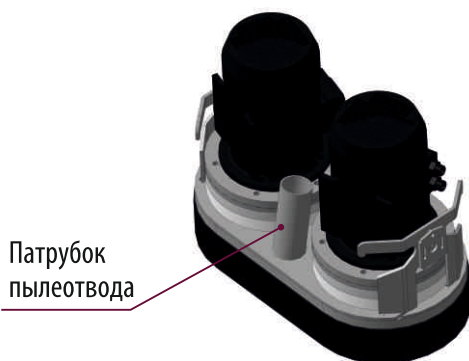
Рис. 3 Подсоединение пылесоса
