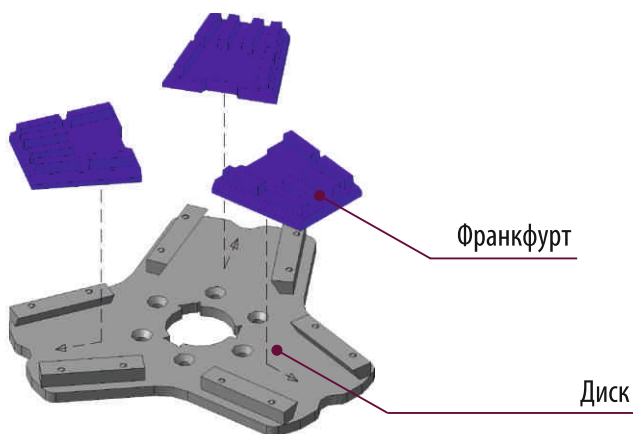
Рис. 9 Установка алмазных франкфуртов
