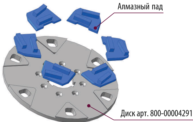
Рис. 8 Установка алмазных падов
